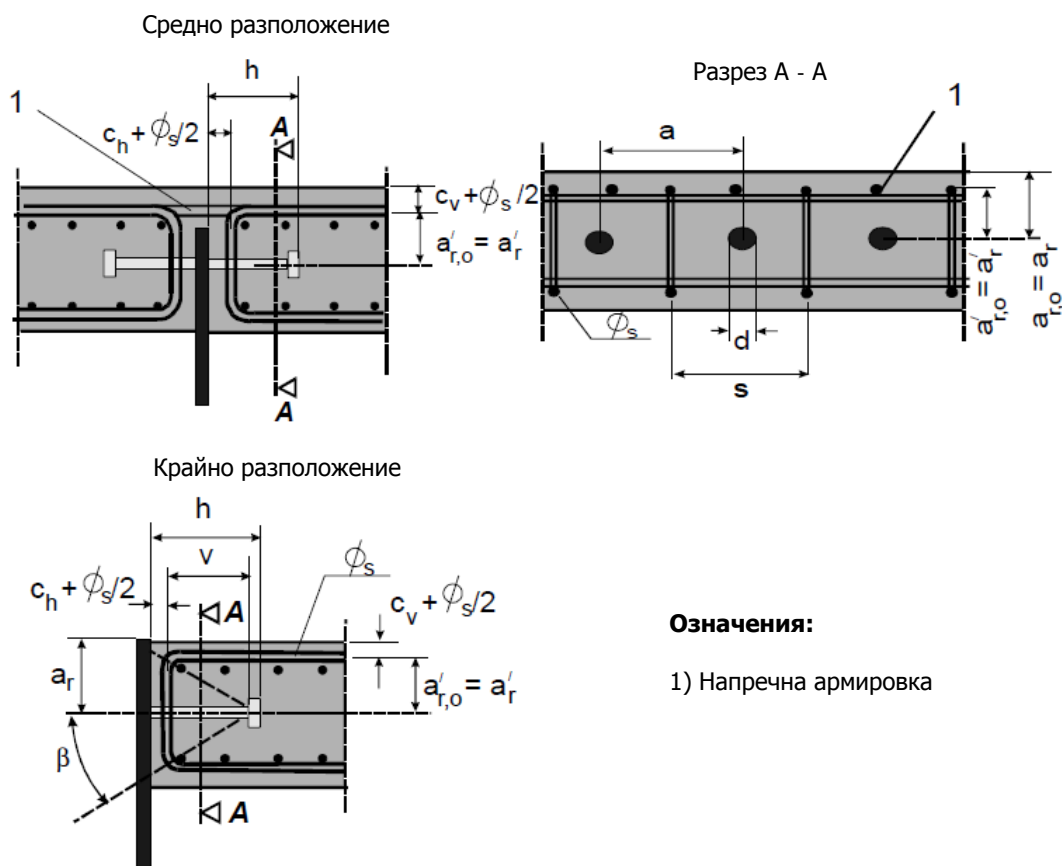
Фигура С.1 – Положение и геометрични размери на дюбелни съединения с хоризонтално разположени дюбели
